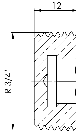
Ansicht / view A-A
