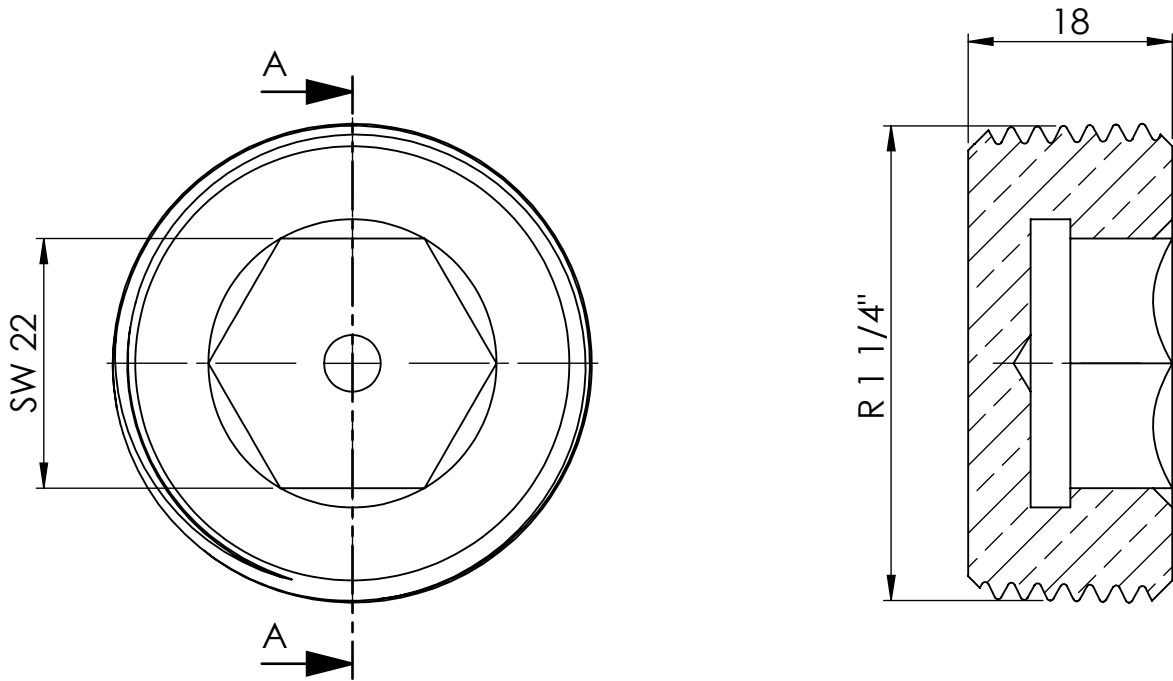
Ansicht / view A-A
