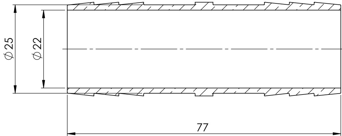
SCHNITT A-A
