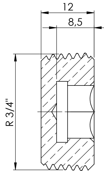
Ansicht / view A-A
