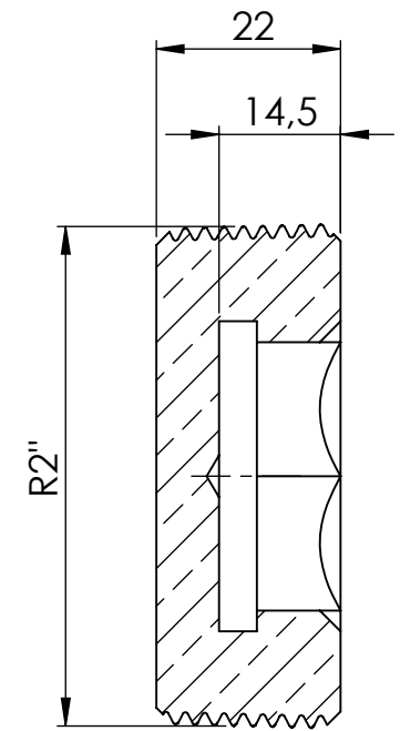
Ansicht / view A-A
