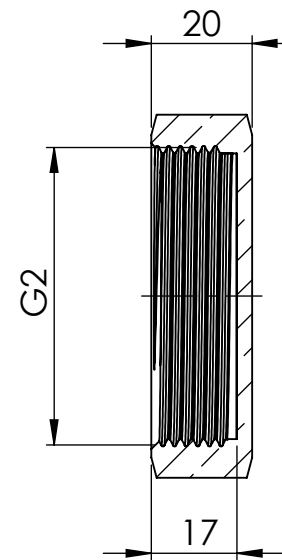
SCHNITT A-A
