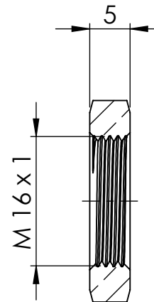
SCHNITT A-A
