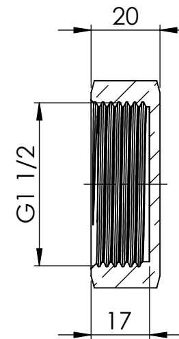
SCHNITT A-A
